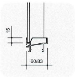
PROFILIT enkelwandig
