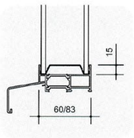
PROFILIT dubbelwandig
