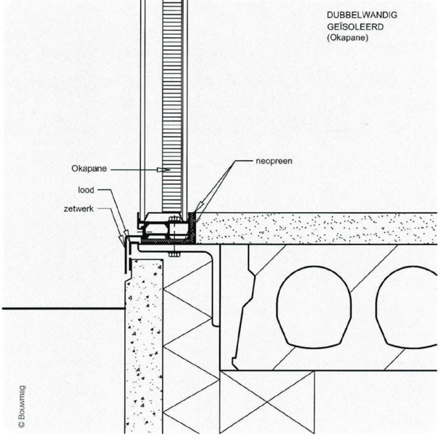
PROFILIT dubbelwandig
